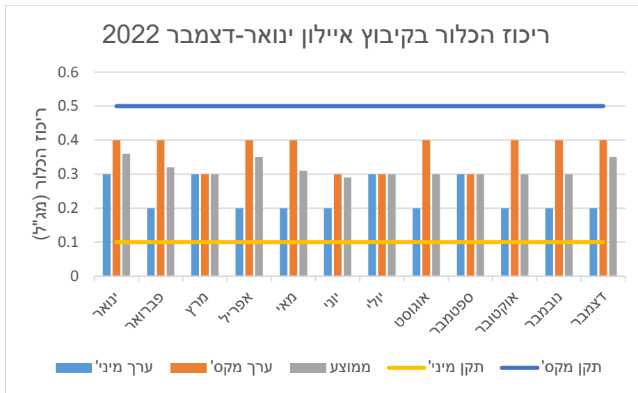
גרף 1 - ריכוזי הכלור ברשת
