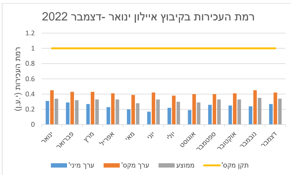
גרף 2 - רמת העכירות ברשת
